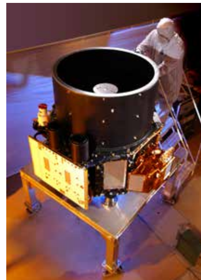
CALIPSO
